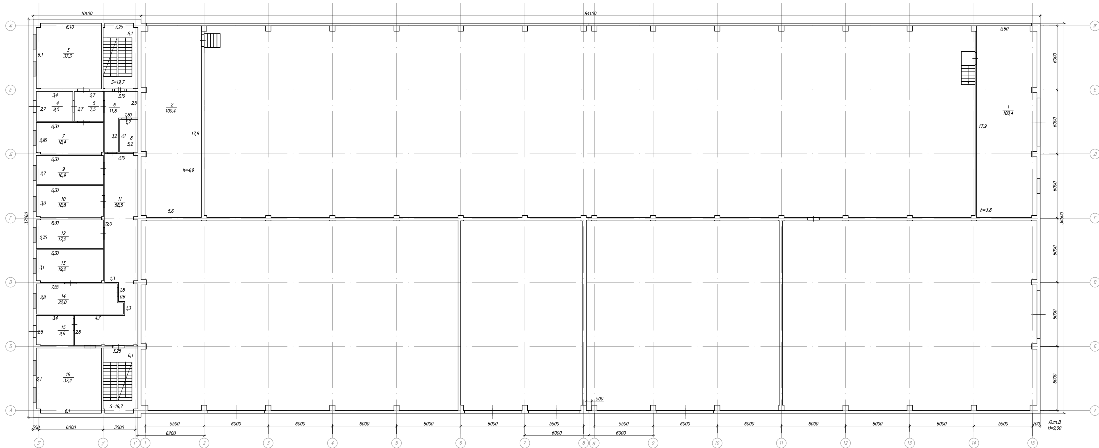
План 2-го этажа S=529,3м 2
