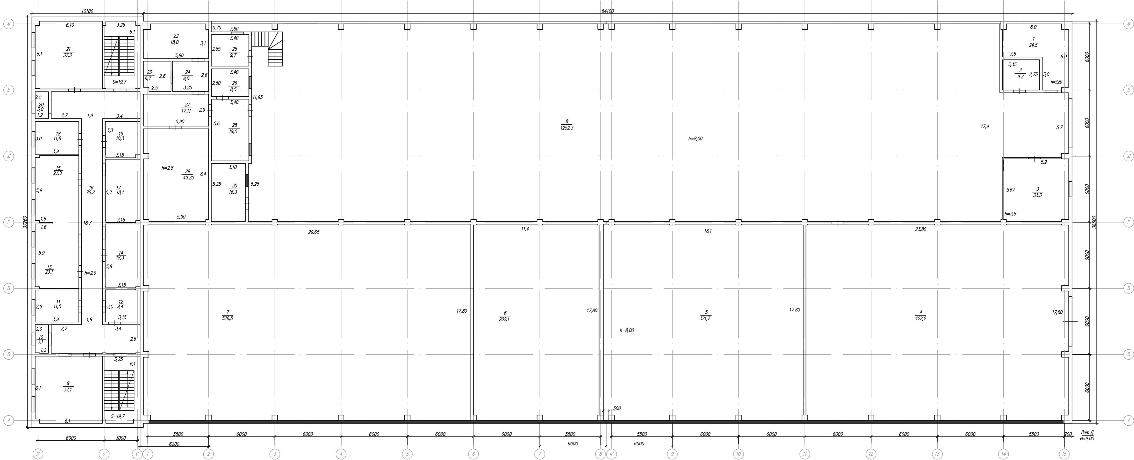
План 1-го этажа S=3291,0м 2
